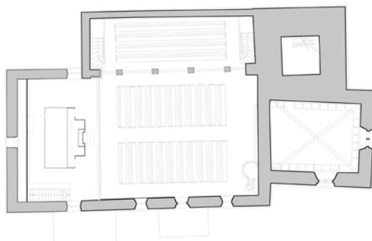
Niveau tribune
