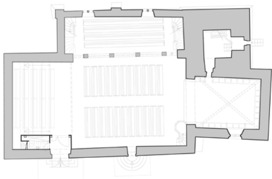
Niveau estrade
